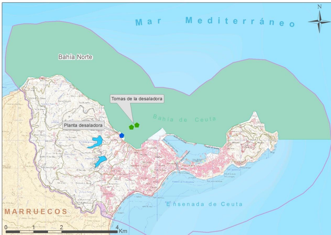
Figura 11. Ubicación de la planta desalinizadora de agua de mar.
